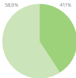
Energieträgermix Ökostrom-Produkte
