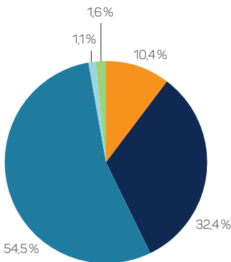
Gesamtenenergieträgermix* EWB
