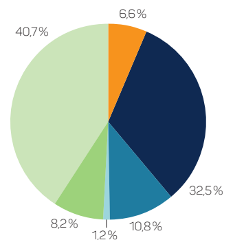
Energieträgermix Deutschland
