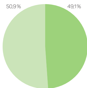
Energieträgermix Ökostrom-Produkte
