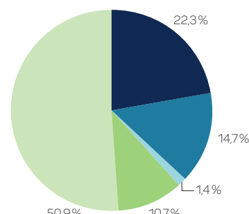
Energieträgermix Deutschland
