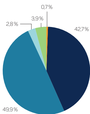
Gesamtenergieträgermix* EWB
