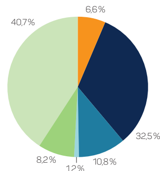
Energieträgermix Deutschland
